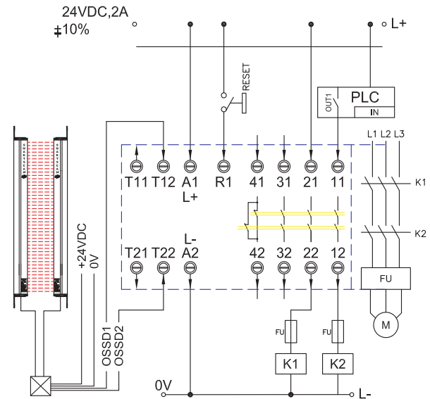
安全光幕
