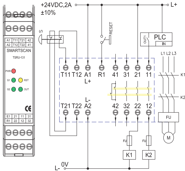
急停按鈕與安全門
