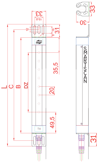
NF2 規格尺寸圖
