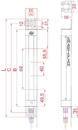
NF3 規格尺寸圖
