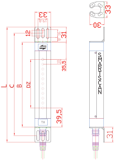
NF1 規格尺寸圖
