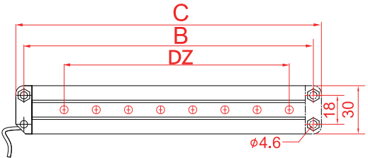
標準型 直接出線 雙孔固定
