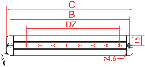
選擇型 C型 直接出線 單孔固定
