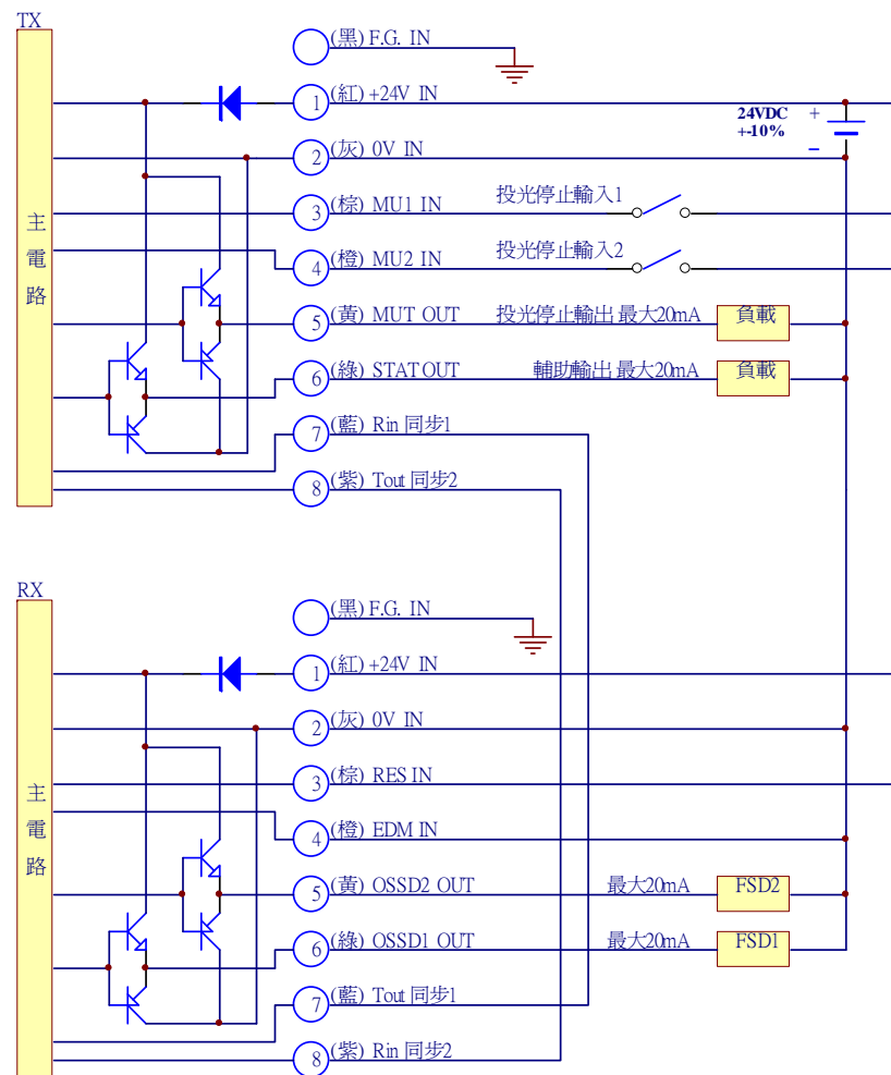
使用 MUTE (靜默)功能之線路圖
